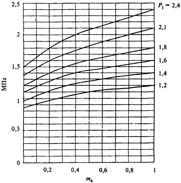
График для определения давления в изотермическом резервуаре в конце выпуска расчетного количества двуокиси углерода
