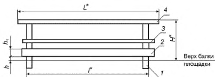
Рисунок В.2 — Ограждение площадок
